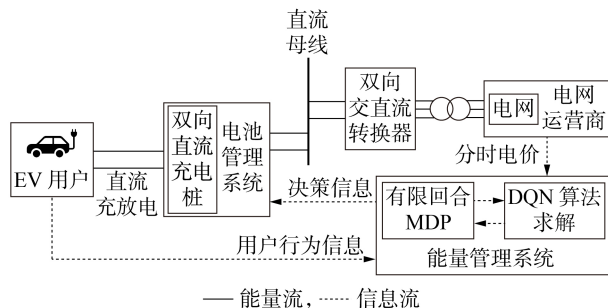
图 1 EVCS 的结构示意图
