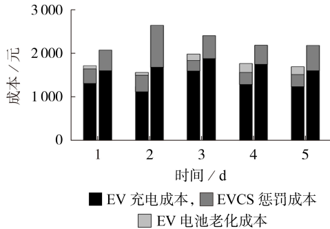
图3 本文策略和RND策略下的日运营成本比较
