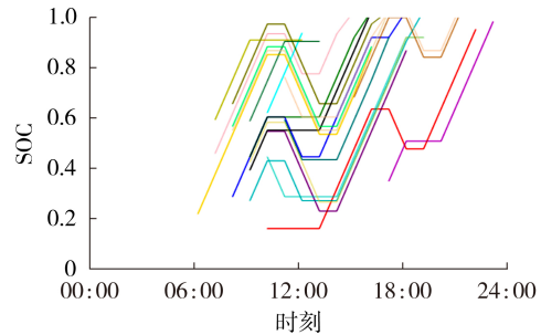
图4 本文策略下20辆EV的SOC变化曲线
