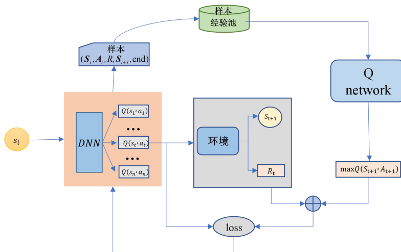
图 A3 DQN 算法结构
