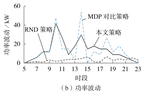
图5 不同的策略下20辆EV的充放电功率比较
