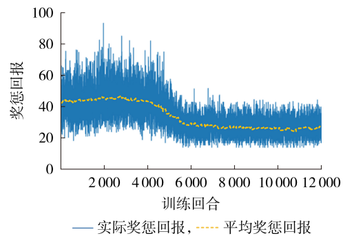
图2 MDP模型的训练结果
